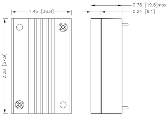
43QAE40-□□S□□U –HS2 7G-0031B-F
