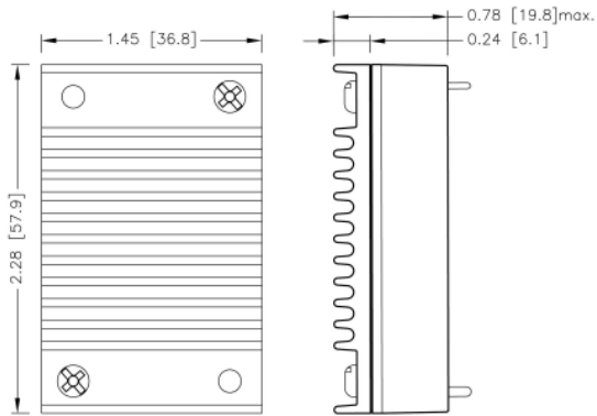
43QAE40-□□S□□0U –HS 7G-0029B-F
